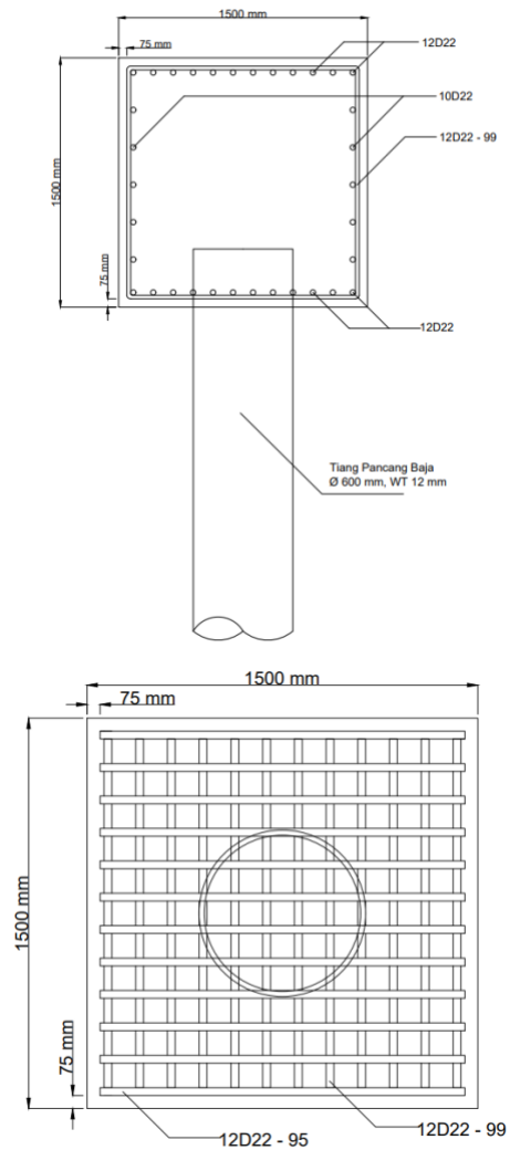
Gambar 5 Desain Penulangan Pile Cap Balok Dermaga
