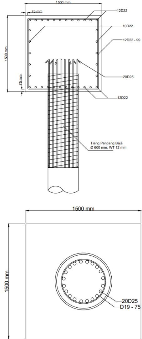
Gambar 7 Desain Penulangan Dowel dan Spiral Pile Cap Balok Dermaga
