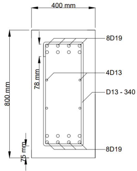
Gambar 9 Desain Penulangan Balok I Trestle
