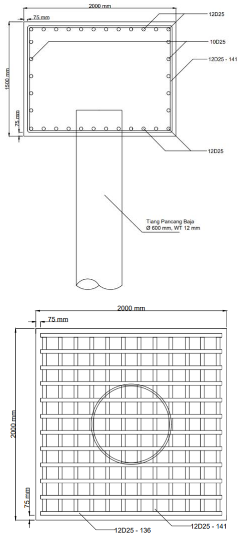
Gambar 6 Desain Penulangan Pile Cap Fender
