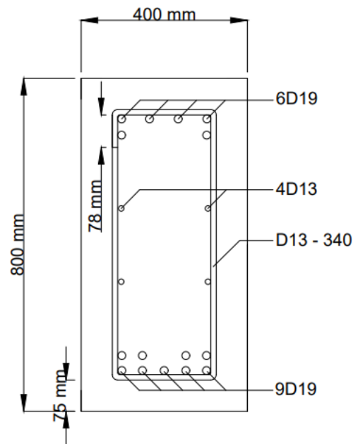
Gambar 10 Desain Penulangan Balok II Trestle
